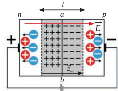
Рисунок 3.32. Обратный переход
