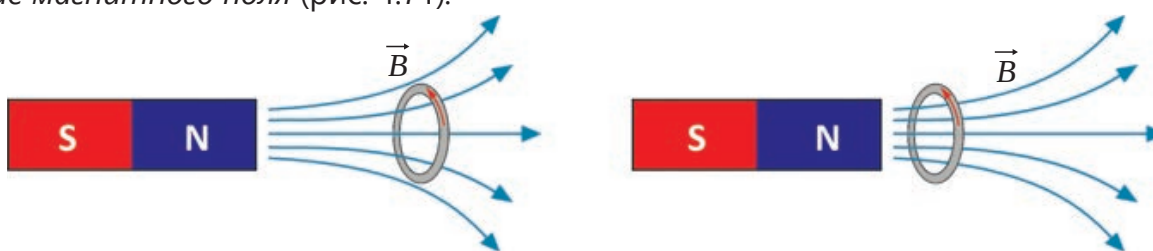
Рисунок 4.71. Изменение магнитного поля означает изменение числа индукционных линий
