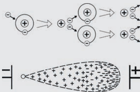
Электропроводность газов
