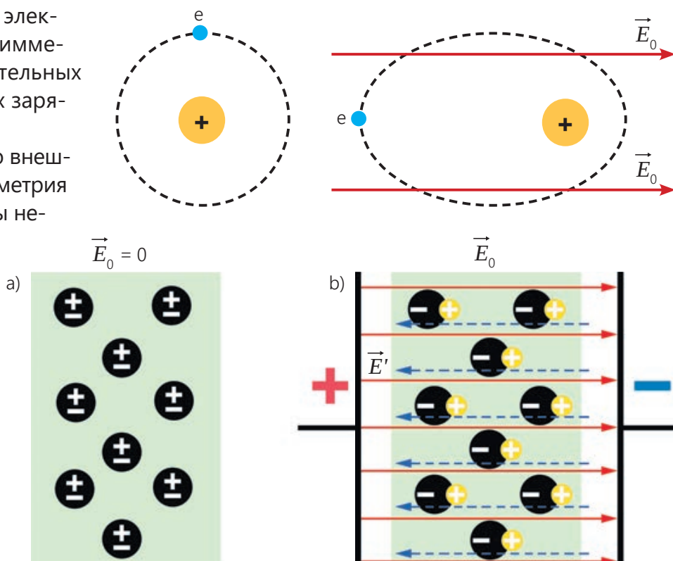
Рисунок 3.4. Неполярный диэлектрик
