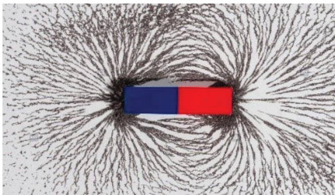
Магнитный спектр
