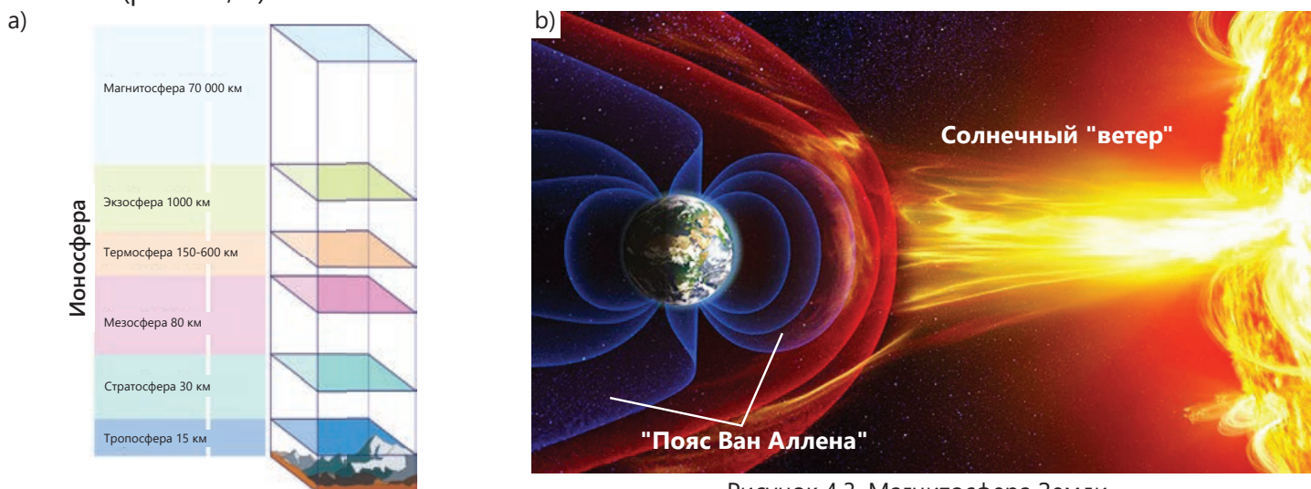
Рисунок 4.3. Магнитосфера Земли
