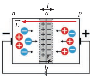
Рисунок 3.31. Прямой переход
