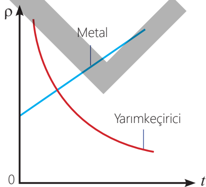
Şəkil 3.24. Xüsusi müqavimət–temperatur qrafiki
