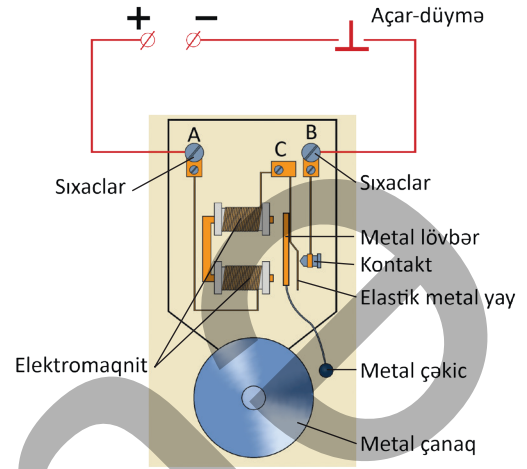
Şəkil 4.35. Elektrik zənginin prinsipial sxemi
