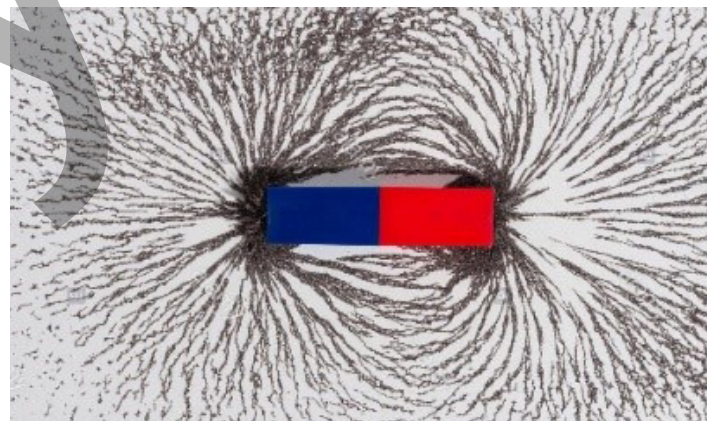
Maqnit spektri
