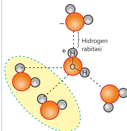
▲ Su molekulunun quruluşu
