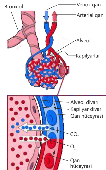
▲ Məməlilərdə qazlar mübadiləsi (oxlar hərəkət istiqamətini göstərir)
