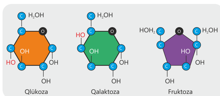
▲ Qlükoza, qalaktoza və fruktozanın quruluşları
